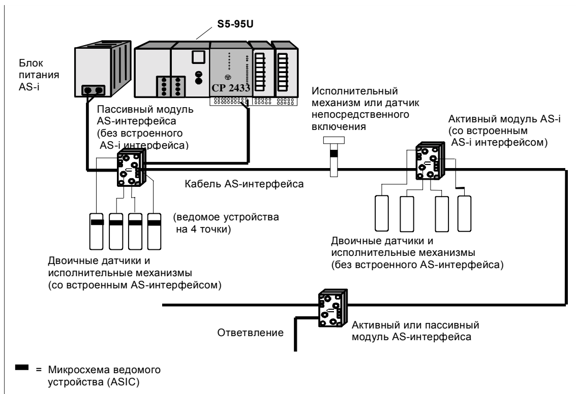
Рисунок 2-5 Пример использования ПЛК SIMATIC S5 с процессором CP 2433
