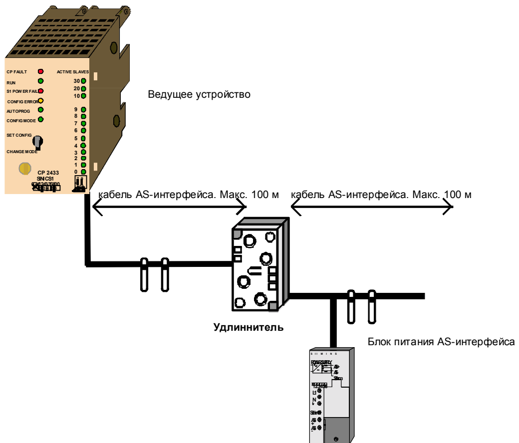
Рисунок 3-6 Использование удлинителя
