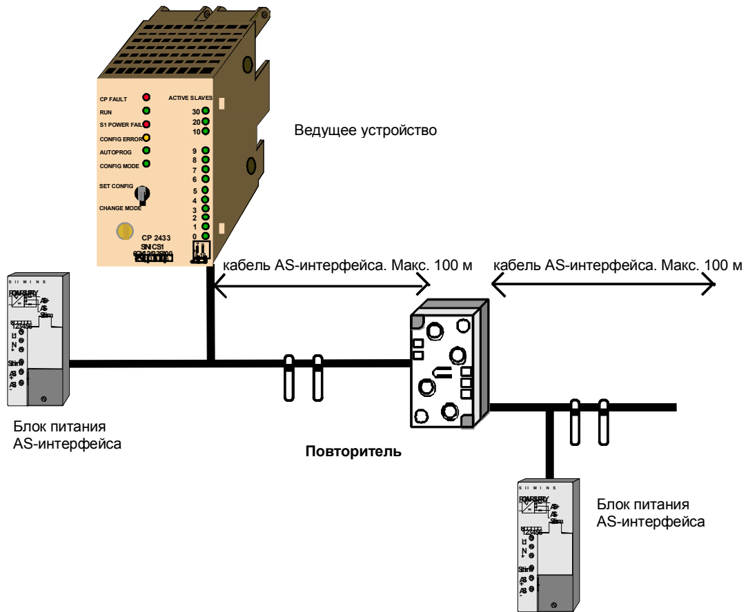
Рисунок 3–5 Использование повторителя
